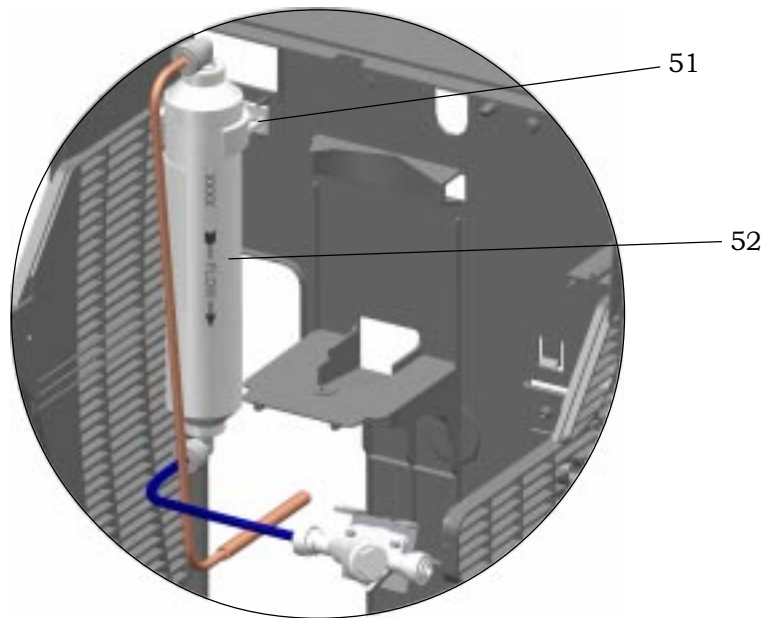
Filter Installation Detail Detalle de la Filtro Instalación Description de Installation del Filtre (Some parts hidden for clarity) (Algunas piezas ocultadas para la claridad) (Quelques pièces cachées pour la clarté)
